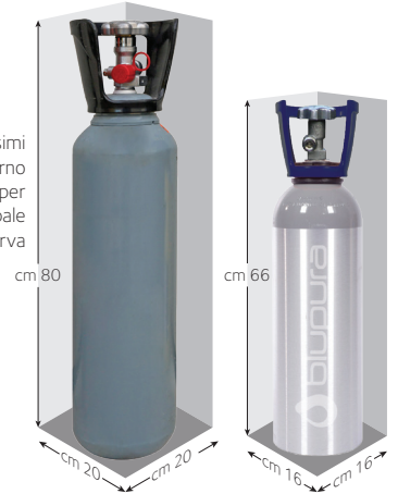
Bombola principale
